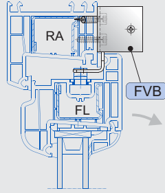
2 RM, 内开窗
